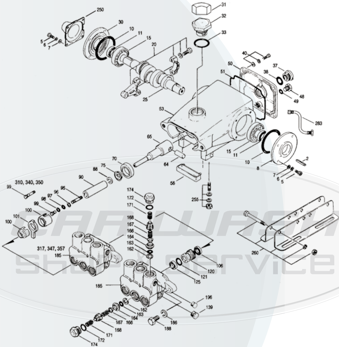
Compressore pompa 350
